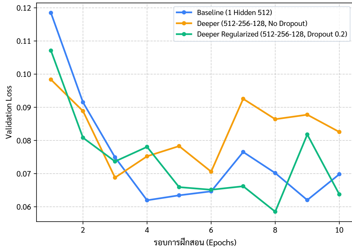
Validation Loss เปรียบเทียบตามสถาปัตยกรรม
