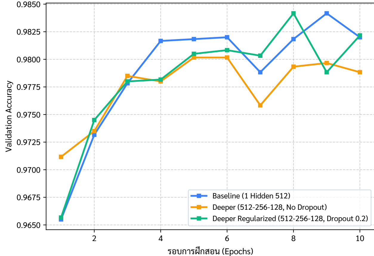
Validation Accuracy เปรียบเทียบตามสถาปัตยกรรม
